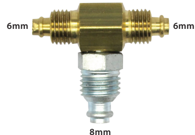
TE DE REDE - 8mm X 6mm
