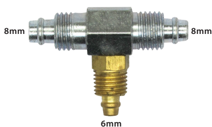
TE DE REDE - 6mm X 8mm
